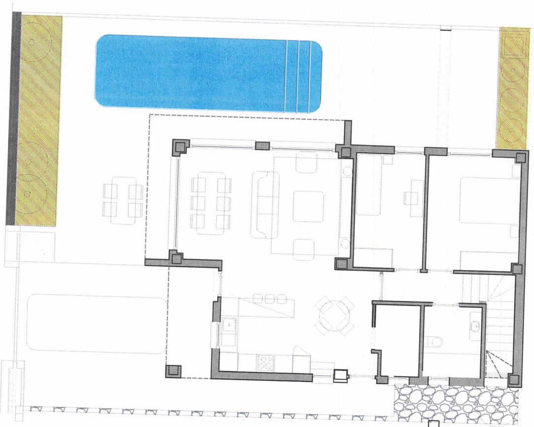
PLANTA BAJA
